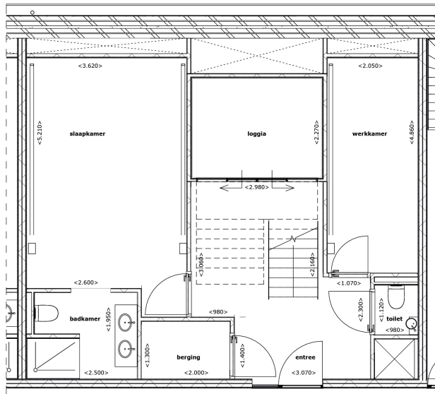
Plattegrond verdieping 03 1:50
