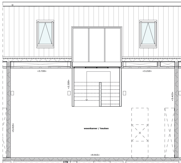
Plattegrond verdieping 04 1:50
